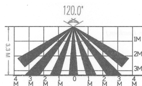
Deckenmontage
