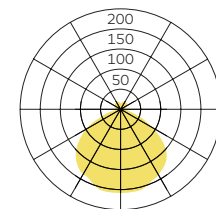
arba Tischleuchte η=82% cd/1000lm
