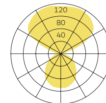
arba Pendelleuchte (500) η=87,9% cd/1000lm
