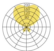
twilight (8027-8040) 79lm/W@4000K
