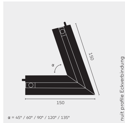
nuit profile - aufbau
