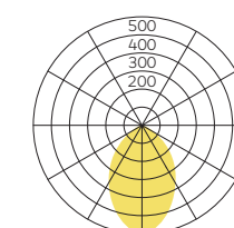
Abstrahlwinkel zwischen 40° und 80° umschaltbar
